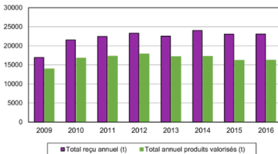
Figure 90 : Evolution annuelle des tonnages du centre de tri depuis 2009 (Source : dip Isséane 2016)
