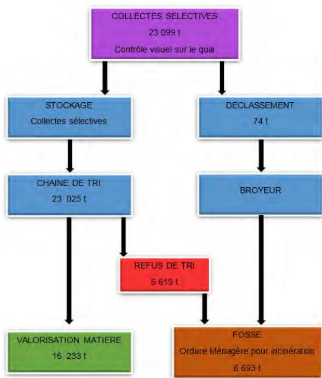
Figure 89 : bilan de matière du Centre de tri (Source : dip Isséane 2016)
