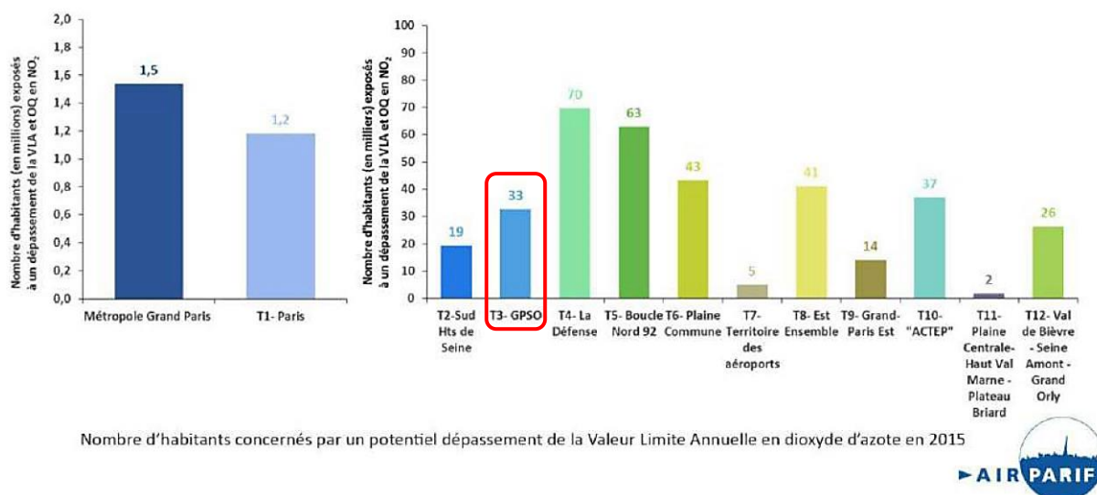
Figure 17 : Nombre d'habitants concernés par un potentiel dépassement de la Valeur Limite Annuelle en dioxyde d'azote en 2015 (Source : prédiagnostic du PCAEM, données AirParif - juillet 2017)
