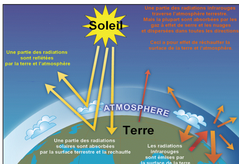
Figure 29 : Vue schématique de l'effet de serre
