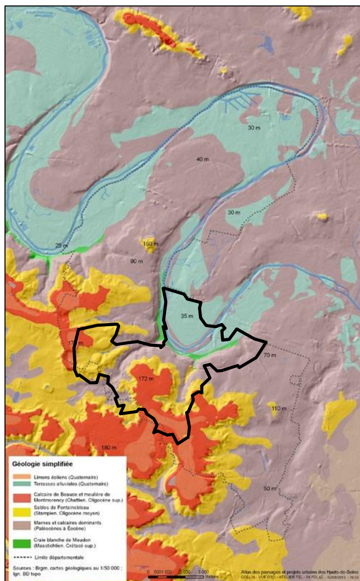
Figure 5 : Carte géologique (Source : Atlas des paysages Hauts de Seine)
