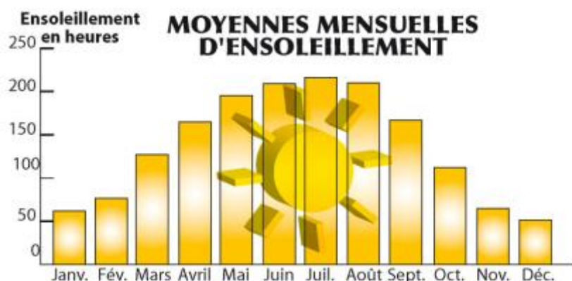
Figure 10 : Moyennes mensuelles d'ensoleillement (Source : CDT Evaluation environnementale GPSO 2012)
