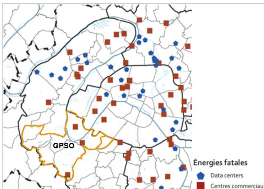
Figure 71 : Recensement des Data Centers. (Source : APUR, étude Paris 2050 Air Energie Climat solaire)
