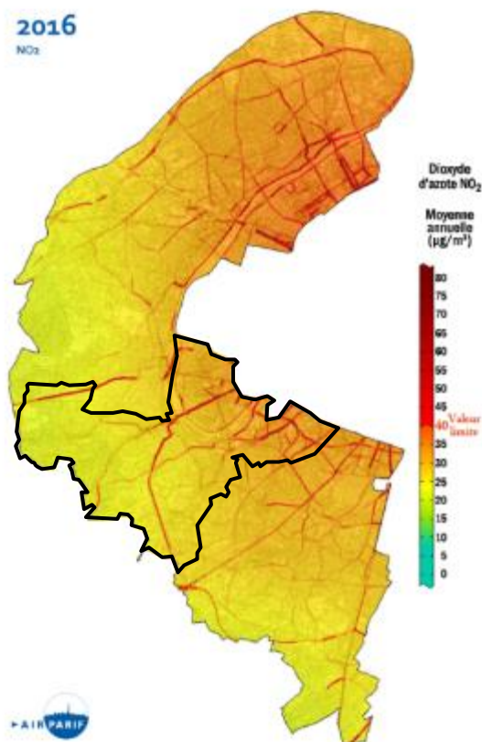
Figure 22 : Concentrations de NO 2 à l'échelle du territoire (Source AirParif-2016)
