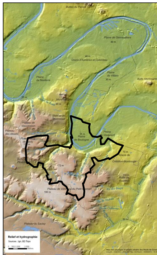
Figure 3 : Carte du relief et hydrographie (Source : Atlas des paysages Hauts de Seine)
