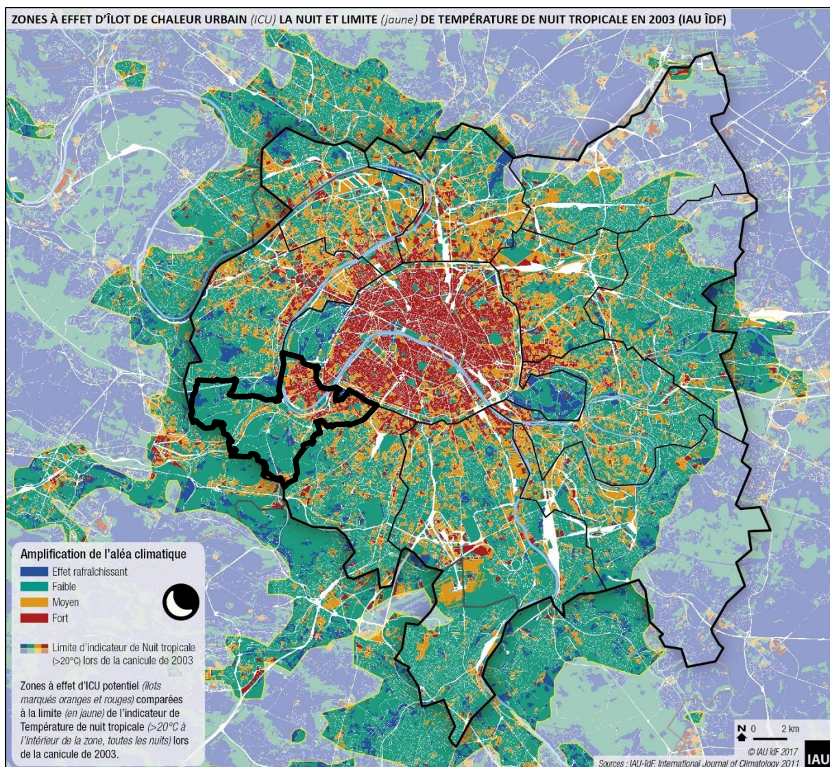
Figure 11 : Représentation des zones à effet de chaleur urbain (Source : IAU)
