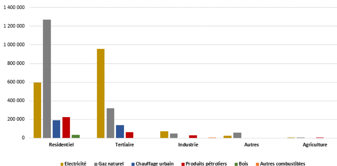
Figure 64 : Consommations d'énergie en MWhEF par secteur et par source d'énergie en 2012, (Source : ROSE, diagnostic énergie du territoire de GPSO)
