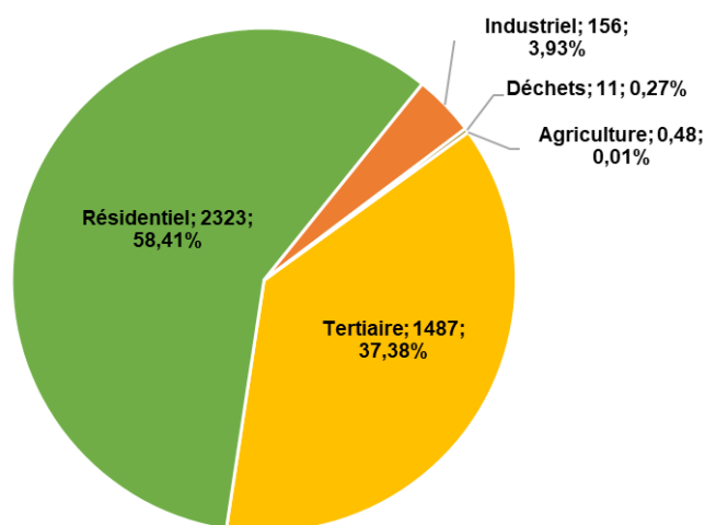
Figure 62 : Répartition des consommations d'énergie en GWhEF par secteur en 2012 (Source : ROSE)
