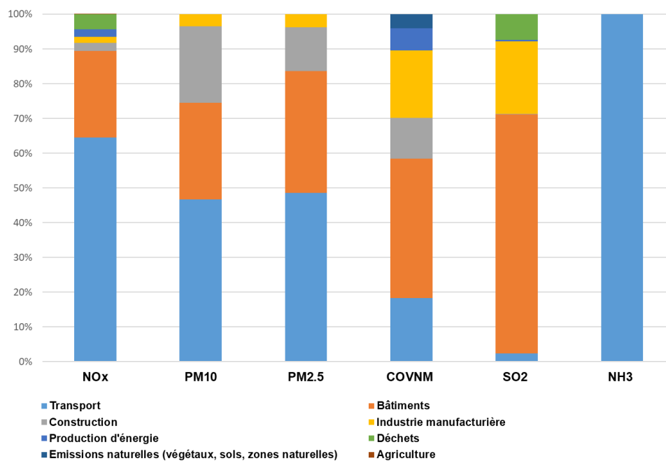
Figure 15 : Répartition des émissions de polluants par secteur
