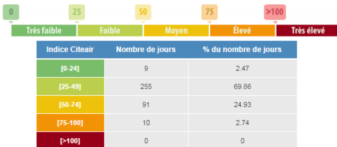
Figure 24 : Répartition annuelle des indices pour le département des Hauts de Seine en 2017 (Source : airparif)
