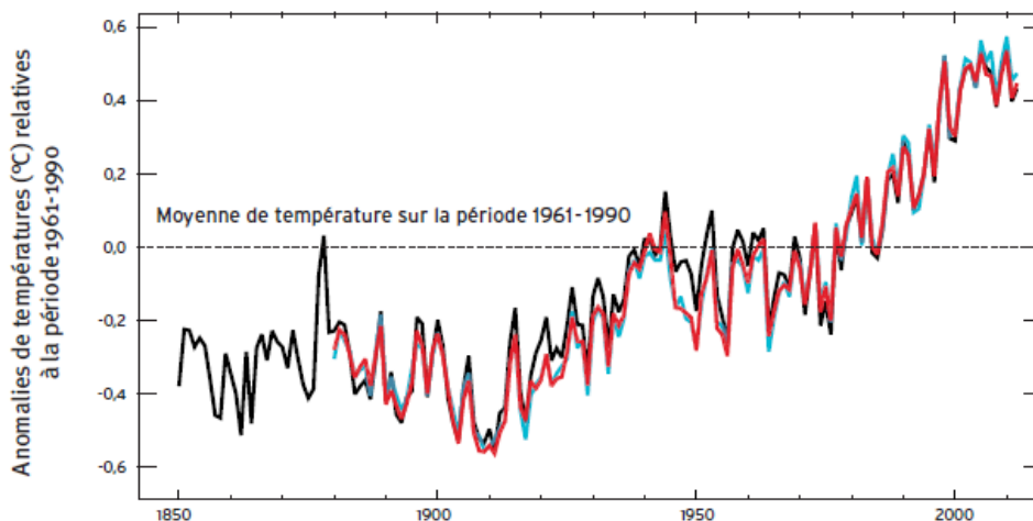
Figure 30 : Anomalies observées de températures moyennes en surface, combinant les terres émergées et les océans, de 1850 à 2012 (Source : Réseau Action Climat : kit pédagogique sur les changements climatiques selon le 5 ème rapport du GIEC 1 er groupe de travail 2013)
