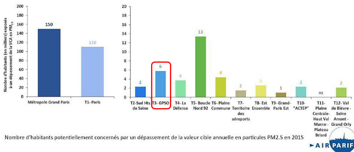
Figure 20 : Nombre d'habitants concernés par un potentiel dépassement de la Valeur Limite Journalière en PM 2.5 en 2015 (Source : prédiagnostic du PCAEM, données AirParif - juillet 2017)
