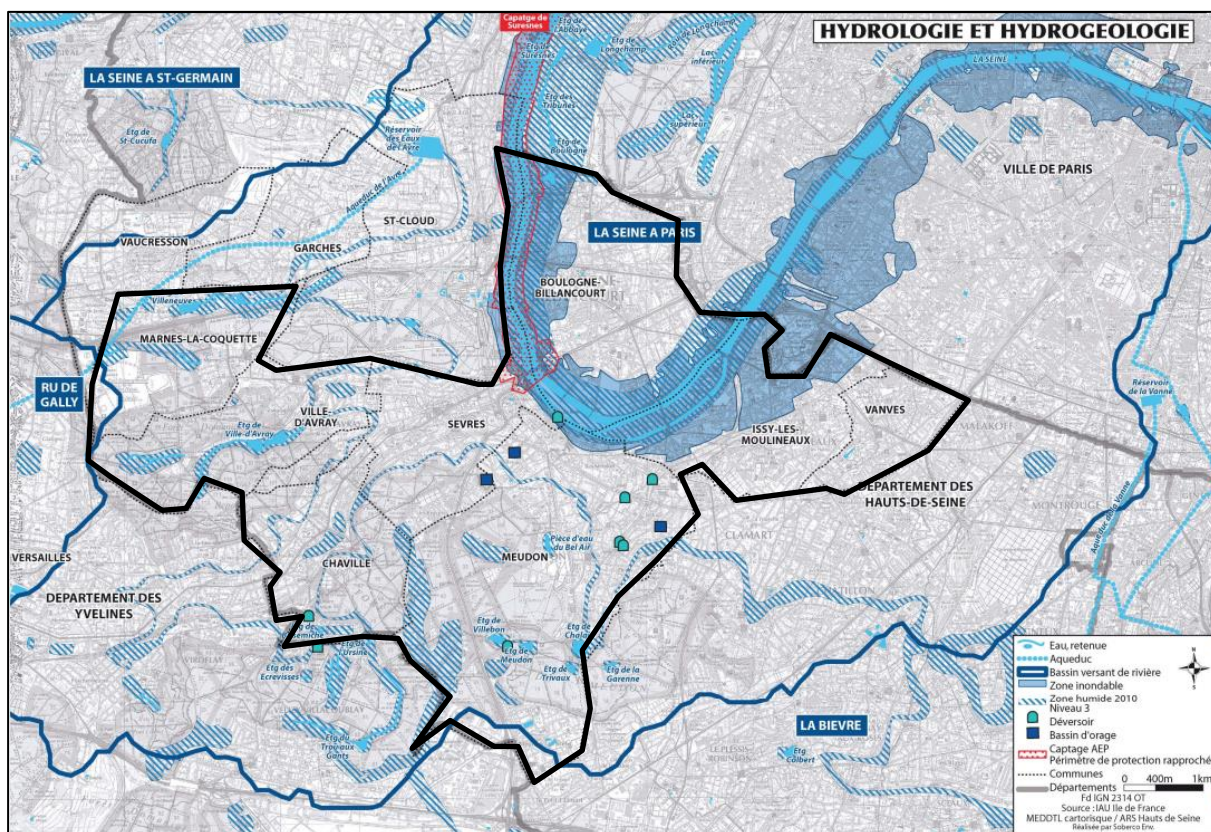
Figure 7 : Hydrologie et hydrogéologie (Source : CDT Evaluation environnementale GPSO 2012)
