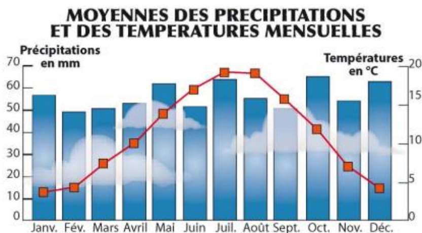
Figure 9 : Moyennes des précipitations et des températures mensuelles (Source : CDT Evaluation environnementale GPSO 2012)
